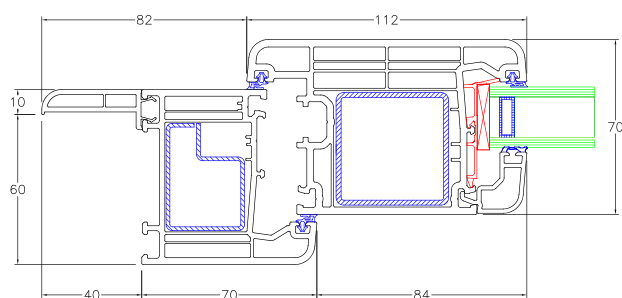
G15/08 Elemento: nodo muro apertura esterna
