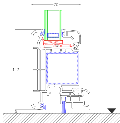
G15/14 Elemento: nodo inferiore apertura esterna
