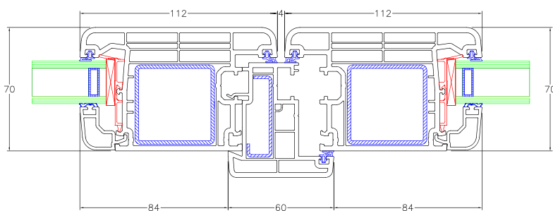
G15/10 Elemento: nodo centrale apertura esterna
