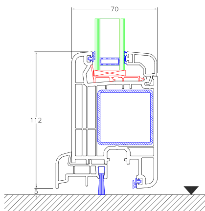
G15/12 Elemento: nodo inferiore apertura interna
