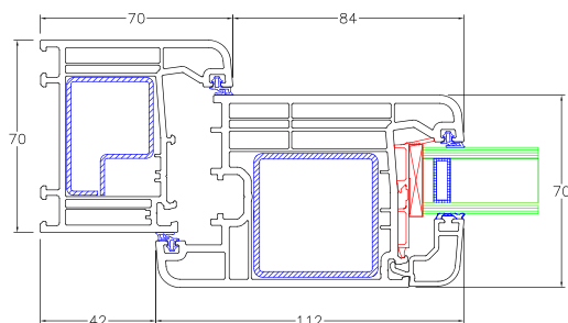
G15/05 Elemento: nodo muro apertura interna (Uf: 1.3 W/MqK)
