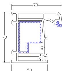
G15/01 Elemento: Telaio L
