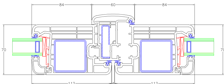
G15/09 Elemento: nodo centrale apertura interna (Uf: 1.3 W/MqK)
