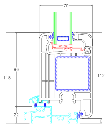
G15/13 Elemento: soglia ribassata apertura interna
