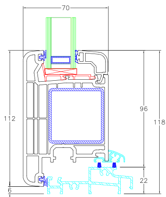
G15/15 Elemento: soglia ribassata apertura esterna
