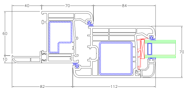
G15/07 Elemento: nodo muro apertura interna
