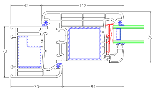
G15/06 Elemento: nodo muro apertura esterna
