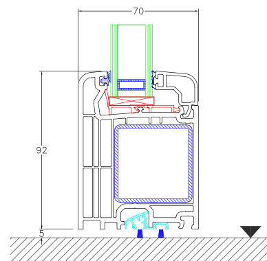
G15/17 Elemento: nodo inferiore porta antipanico
