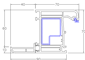
G15/02 Elemento: Telaio Z
